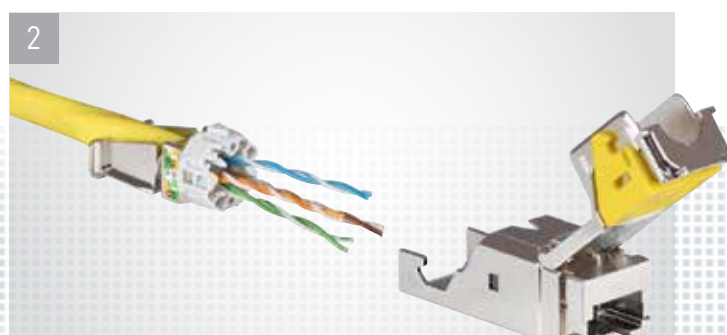
2 Пропустить пары кабеля сзади через основание коннектора
